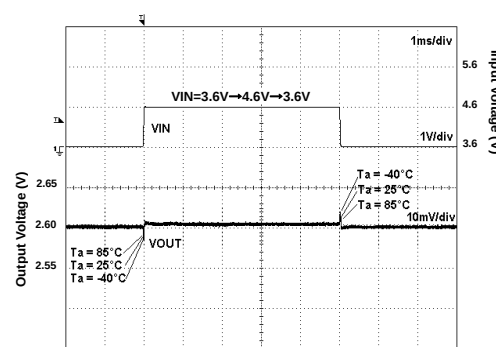
Fig 154. VIN Response
