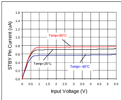
Fig 262. VSTBY - ISTBY
