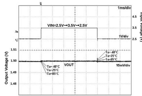
Fig 52. VIN Response
