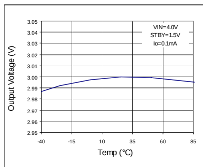
Fig 216. VOUT - Temp
