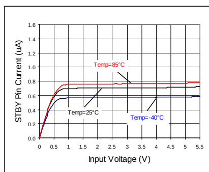
Fig 158. VSTBY - ISTBY
