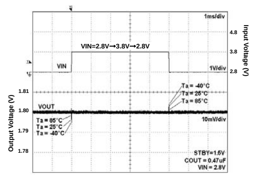
Fig 77. VIN Response
