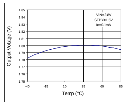
Fig 61. VOUT - Temp
