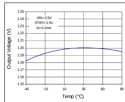
Fig 11. VOUT - Temp
