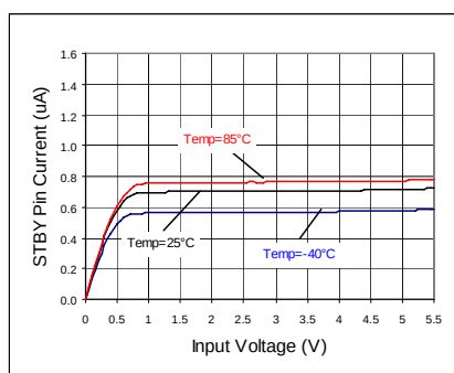
Fig 56. VSTBY - ISTBY
