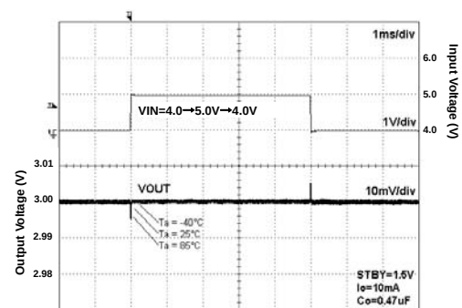
Fig 232. VIN Response
