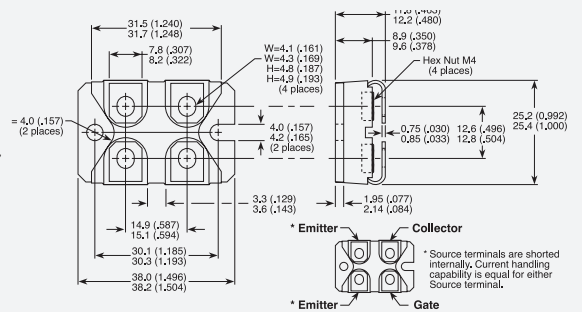
SOT-227
